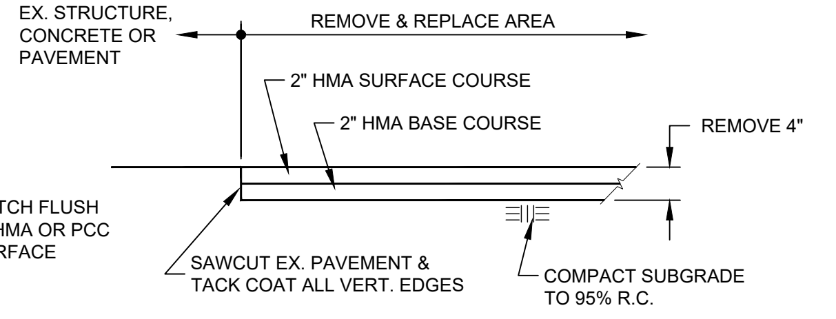
2 REMOVE & REPLACE 4\"/>
