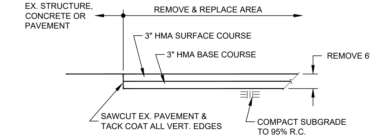
3 REMOVE & REPLACE 6\"/>
