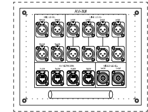
4 AV PANEL AV-A20, A21
